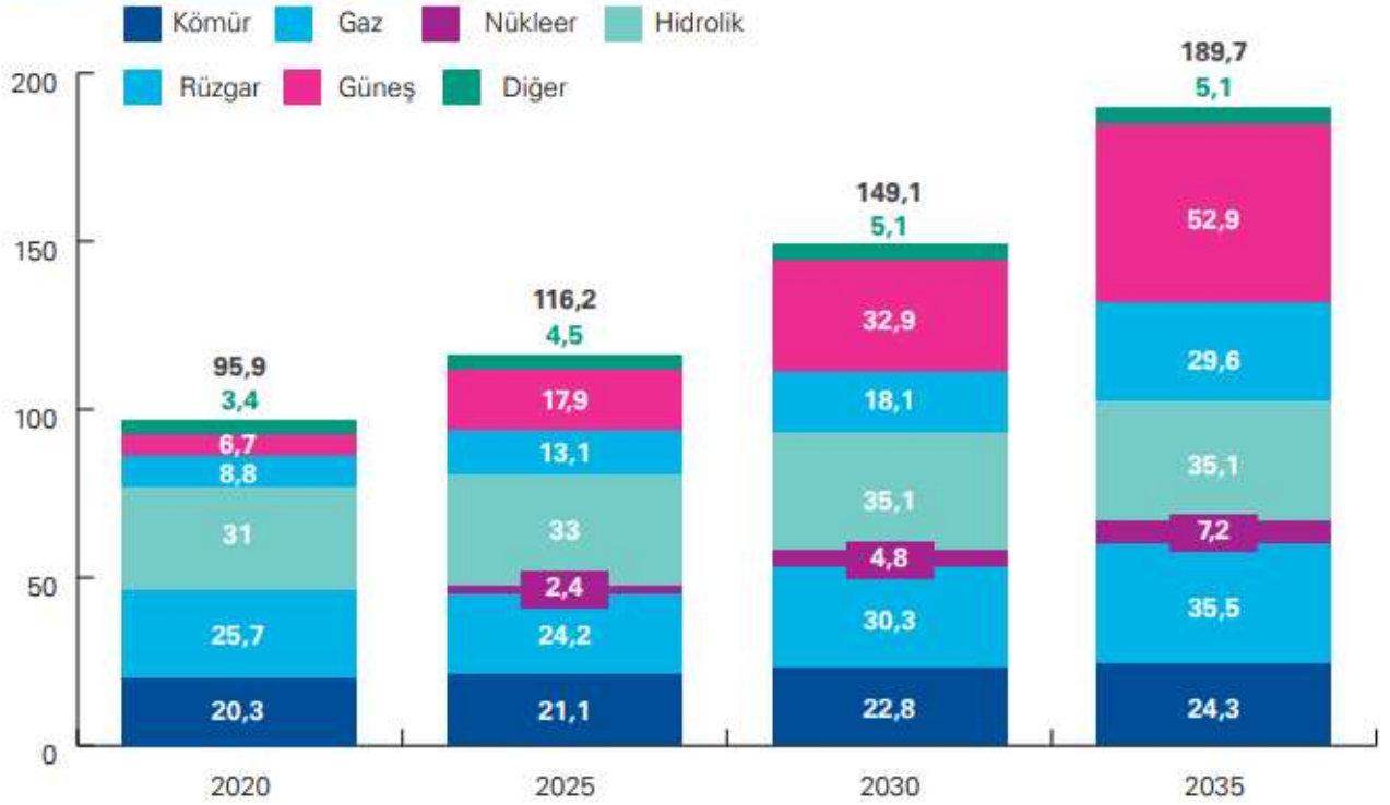
Kaynaklara Göre Kurulu Güç (GW)
